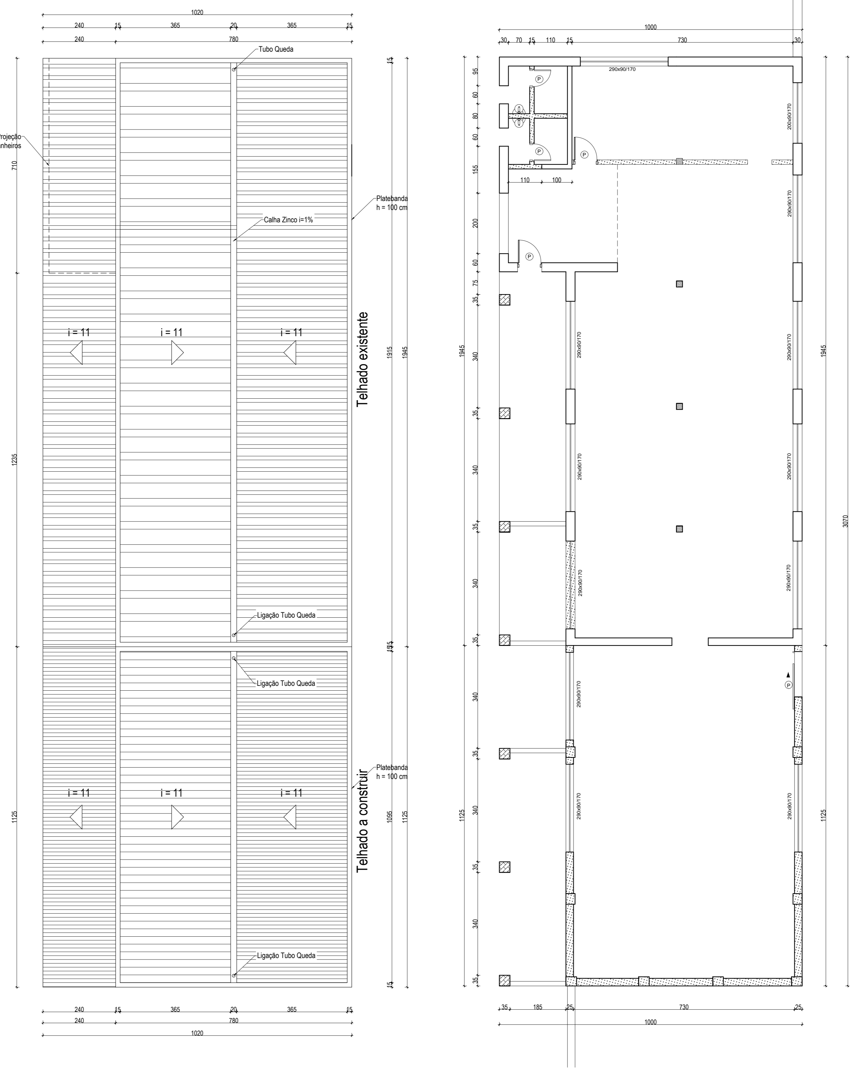
Diagrama Telhado Esc.: 1/75
