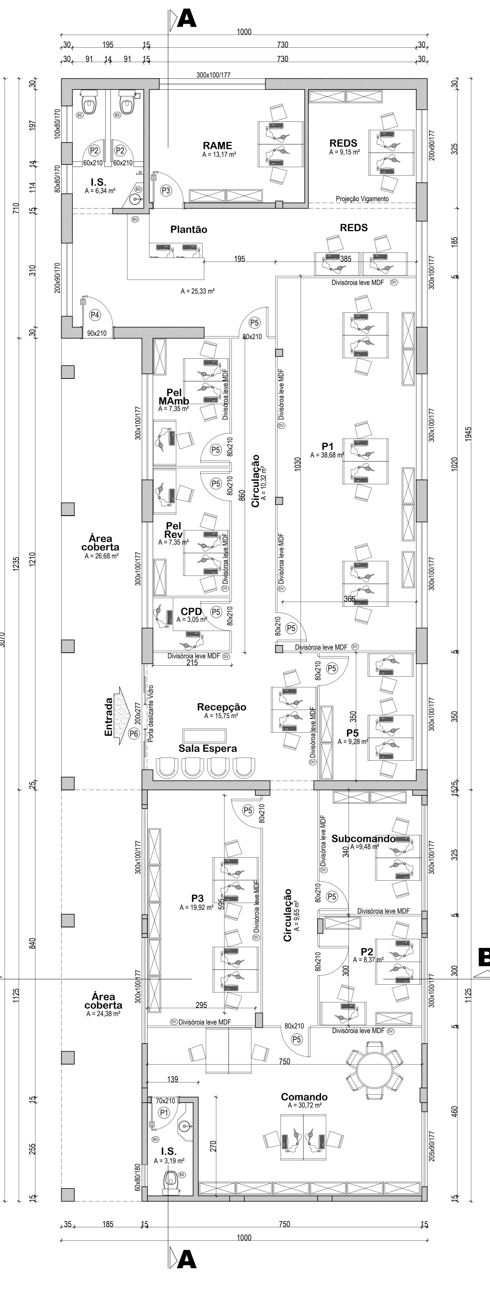
Planta Baixa Layout Esc.: 1/50
